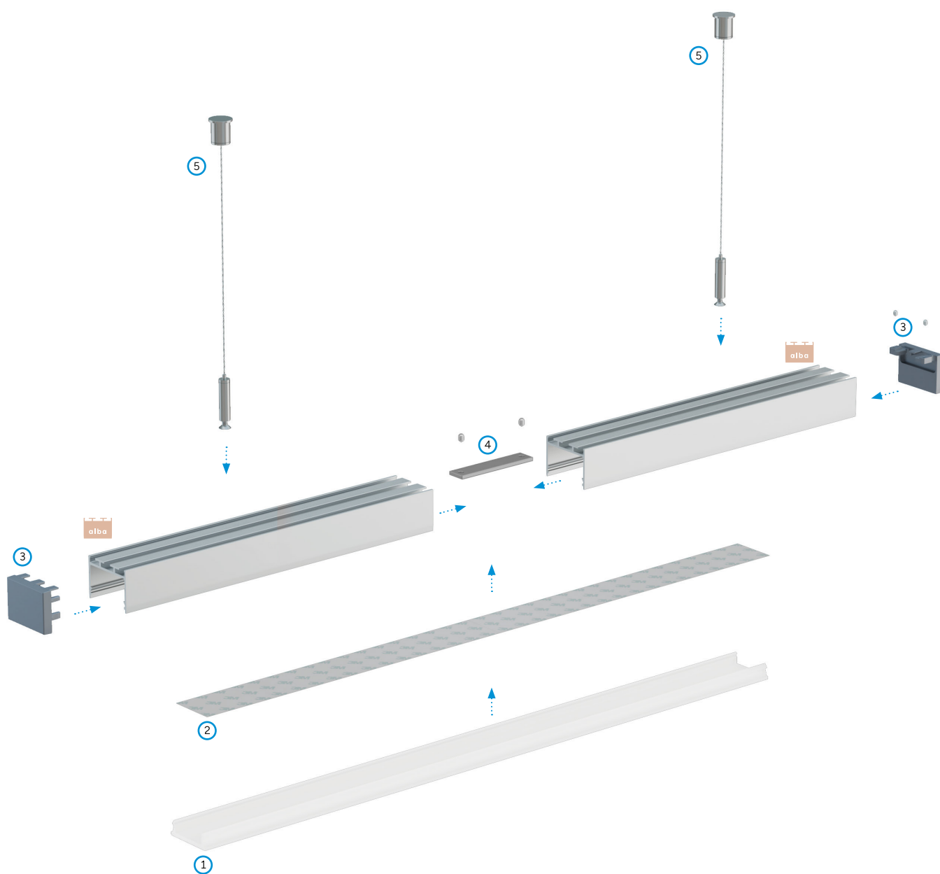
Schemat montażu elementów systemu oświetlenia LED z wykorzystaniem profilu LED alba oraz: (1) klosza midi , (2) dwóch taśm LED , (3) zaślepek bez otworów , (4) łącznika prostego , (5) zawiesi .
